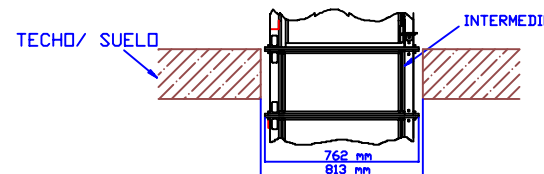
DETALLE "A" (CONFIGURACIÓN ATRAVESANDO SUELO)
